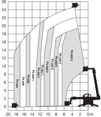
Geschwenkt abgestützt
