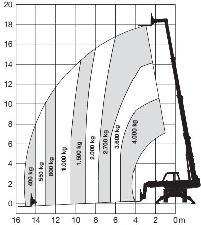
Geschwenkt abgestützt
