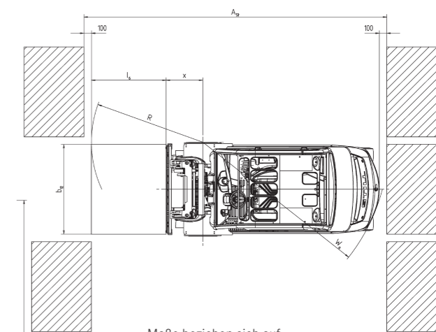
Maße beziehen sich auf senkrecht stehendes Hubgerüst
