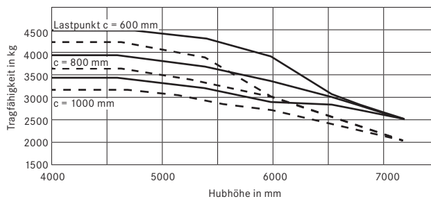
Tragfähigkeiten RX 60-45/600 mit Dreifach-Hubgerüst
