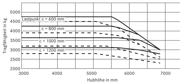
Tragfähigkeiten RX 60-50/600 Dreifach-Hubgerüst ab BH2400
