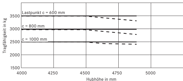
Tragfähigkeiten RX 60-40/600 Tele-Hubgerüst
