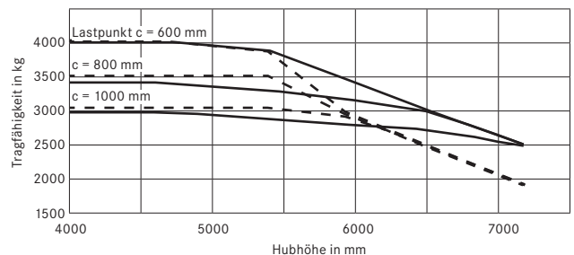
Tragfähigkeiten RX 60-40/600 mit Dreifach-Hubgerüst
