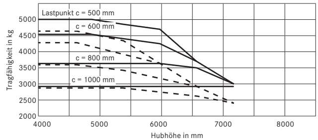
Tragfähigkeiten RX 60-35/600 mit Dreifach-Hubgerüst
