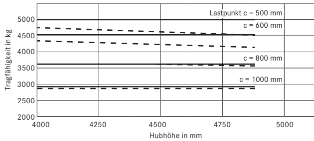
Tragfähigkeiten RX 60-45 Dreifach-Hubgerüst/Zwillingsbereifung
